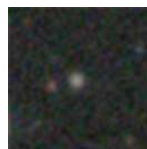
PGC 3869911 – Mag 17.41
