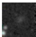
PGC 4013466 – Mag 18.35
