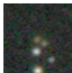
PGC 2083731 – Mag 18.57
