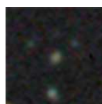
PGC 3501418 – Mag 18.19
