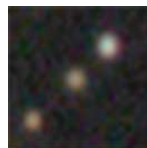
PGC 2072544 – Mag 17.72
