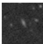
PGC 2082344 – Mag 17.76
