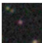
PGC 4007189 – Mag 18.71
