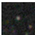
PGC 3388666 – Mag 18.01
