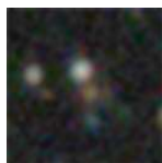
PGC 2095065 – Mag 18.64
