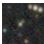
PGC 3501189 – Mag 18.98
