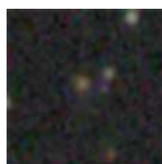
PGC 3501475 – Mag 19.05
