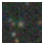
PGC 3501064 – Mag 18.72
