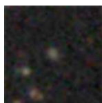
PGC 3501412 – Mag 18.32
