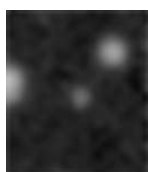
PGC 3501328 – Mag 19.04
