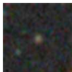
PGC 3501443 – Mag 18.89
