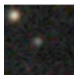
PGC 4007208 – Mag 18.32
