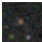
PGC 2083830 – Mag 18.96
