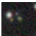
PGC 3688995 – Mag 18.51
