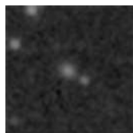
PGC 2094772 – Mag 18.05
