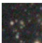
PGC 3501376 – Mag 18.34
