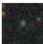
PGC 4007199 – Mag 18.45
