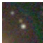
PGC 3501460 – Mag 19.00
