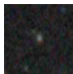
PGC 2071047 – Mag 18.55
