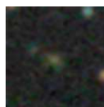
PGC 3388680 – Mag 18.54
