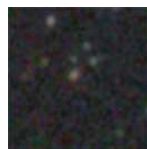
PGC 3501379 – Mag 19.04
