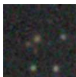
PGC 2074280 – Mag 18.57
