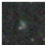
PGC 4007092 – Mag 17.82
