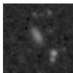
PGC 2096210 – Mag 16.76
