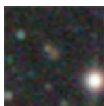
PGC 3501406 – Mag 19.10
