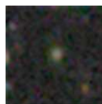
PGC 2092091 – Mag 18.23
