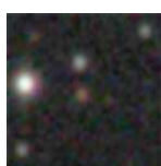
PGC 3501359 – Mag 18.91
