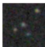
PGC 2074545 – Mag 18.47
