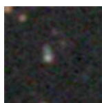
PGC 35001316 – Mag 18.50
